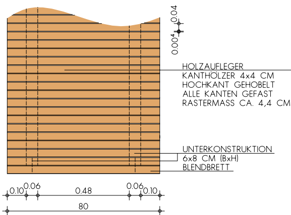
DRAUFSICHT HOLZSTEG
