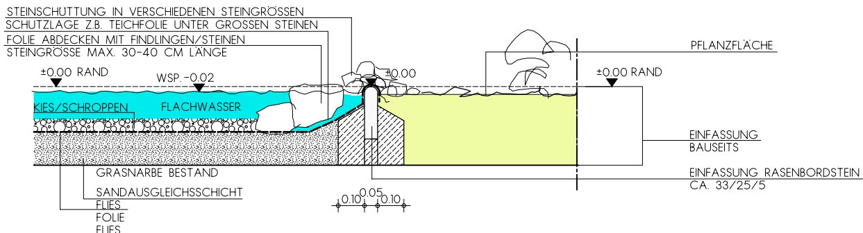
SCHNITT/DETAIL A: SEE-KANTE-KIES SEE/WASSERFLÄCHE
