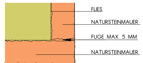
SCHICHT 1 UND 3 DETAIL MAUERECKE
