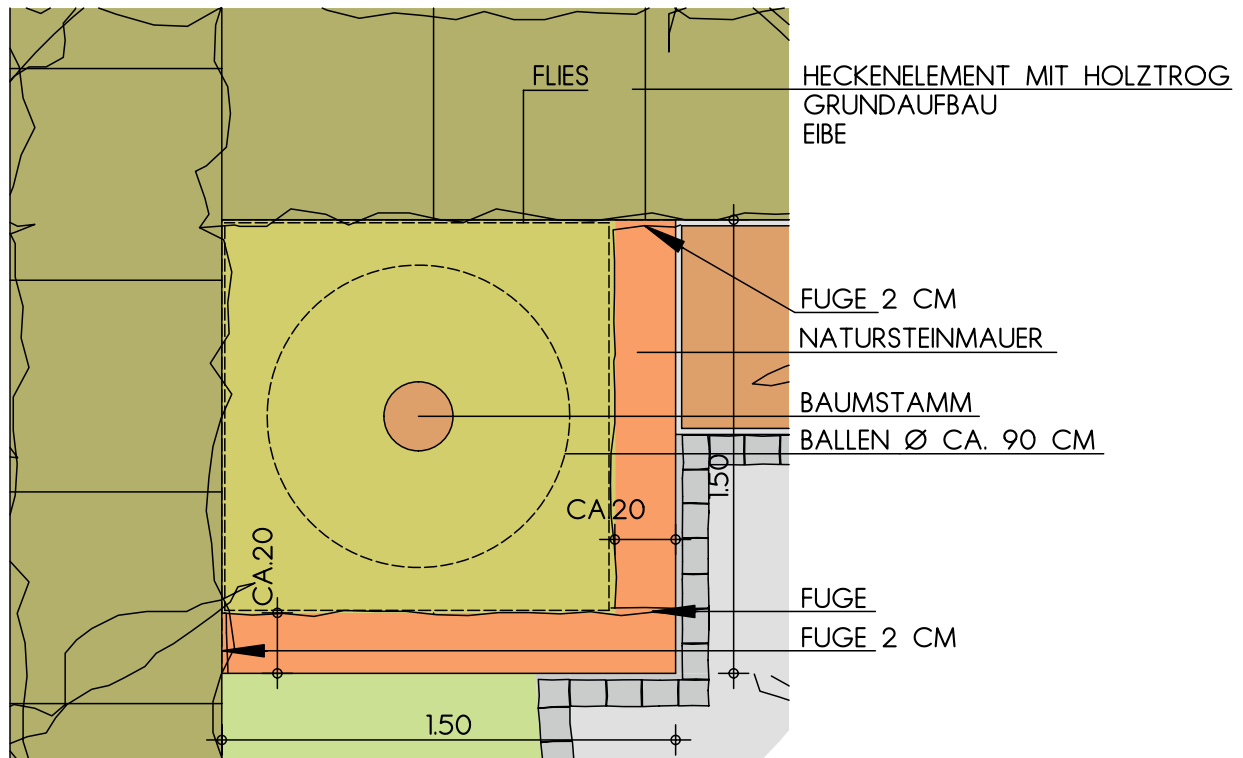
DETAIL SCHICHTENMAUERWERK GRUNDRISS
