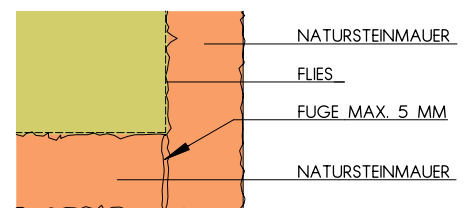
SCHICHT 2 DETAIL MAUERECKE
