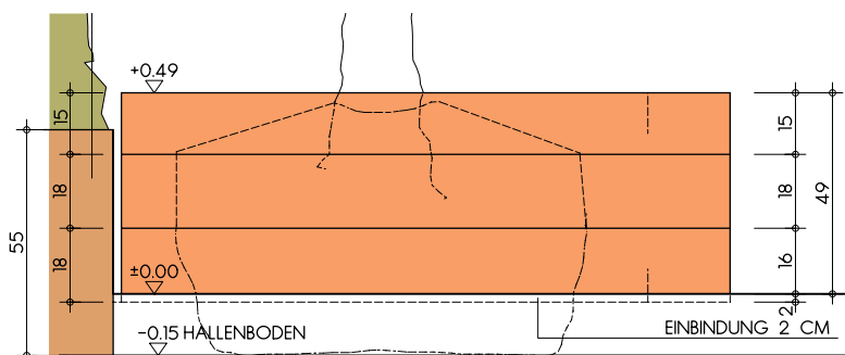
DETAIL SCHICHTENMAUERWERK ANSICHT
