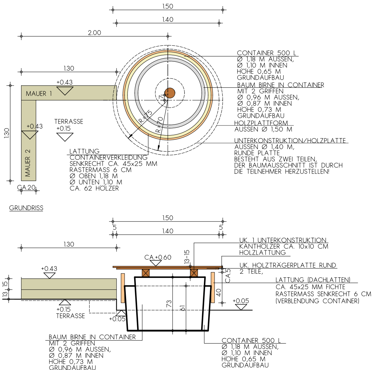
SCHNITT 1-1
